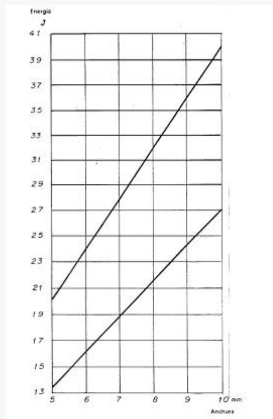
Valor de la energía de rotura mínima (J) para probetas con entalla en V para el ensayo de flexión por choque de anchura comprendida entre 5 mm y 10 mm
