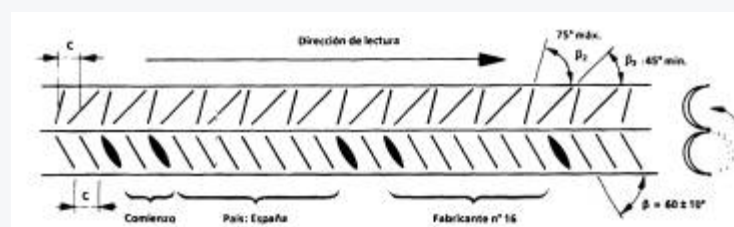
Grabado del tipo de acero B500S
