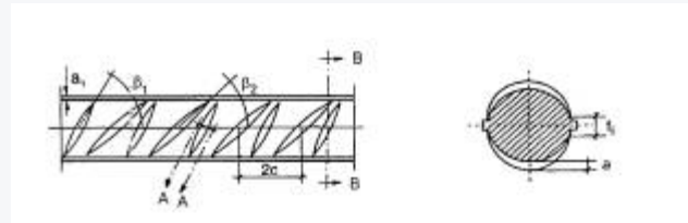
Barra corrugada de acero B500SD
