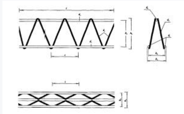
Armadura básica electrosoldada en celosía
