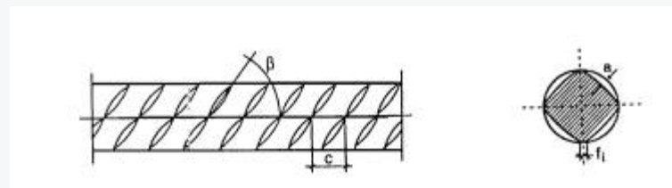
Barra corrugada de acero B500SD
