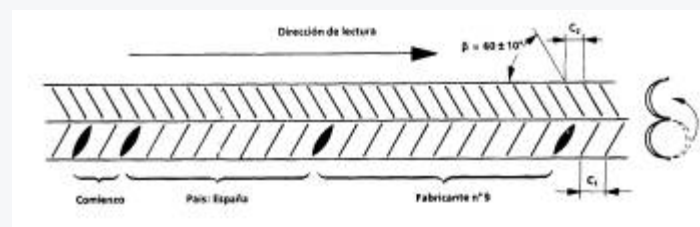
Grabado del tipo de acero B400S
